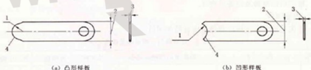
图 2 凸形样板与凹形样板示意图
